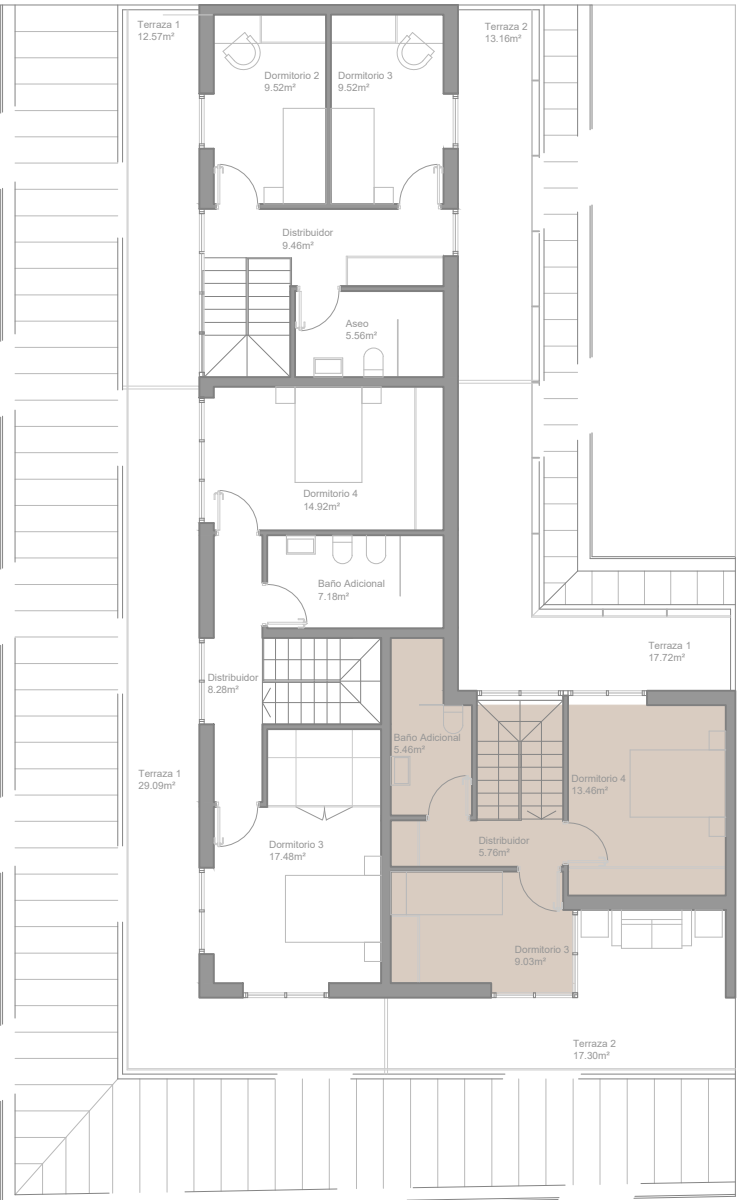
Planta Cuarta - vivienda C - BC
