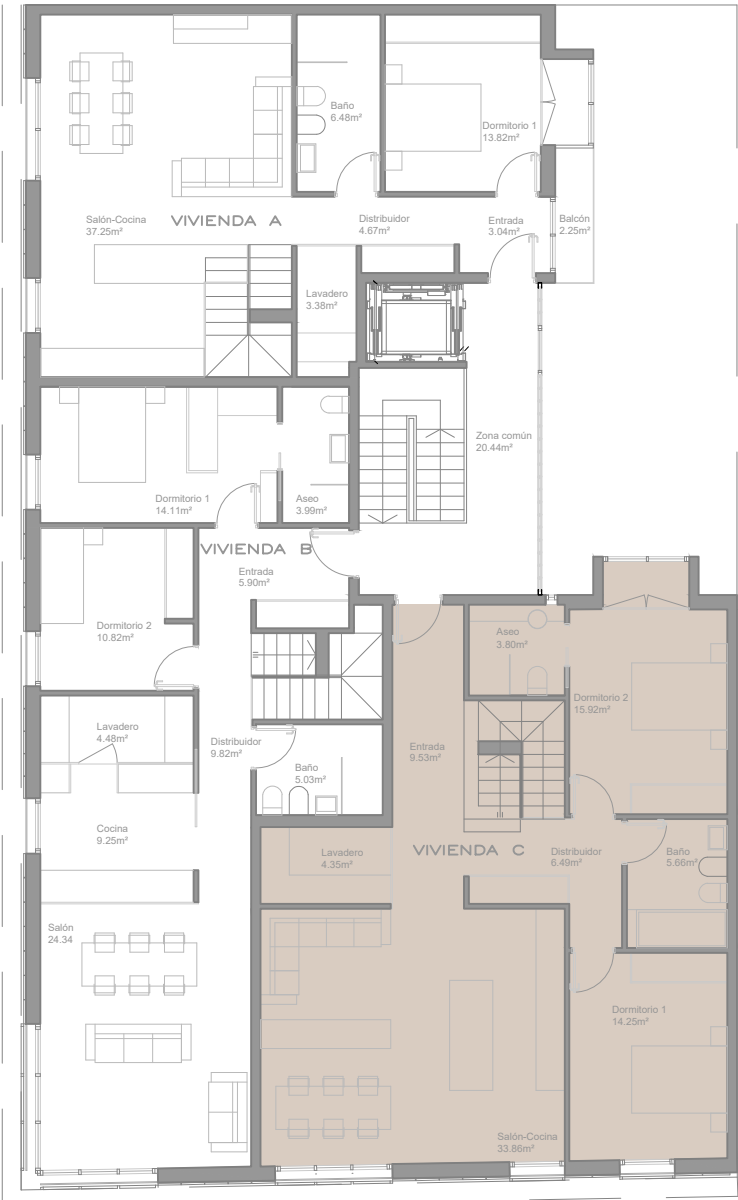
Planta Cuarta - vivienda C
